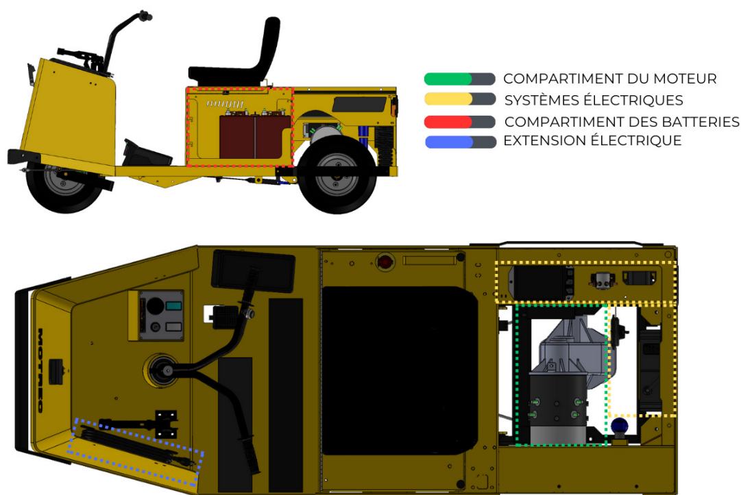
Figure 1. Compartiments des équipements.
