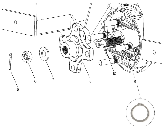
Figure 46. Inspection de l'arbre d'essieu.
