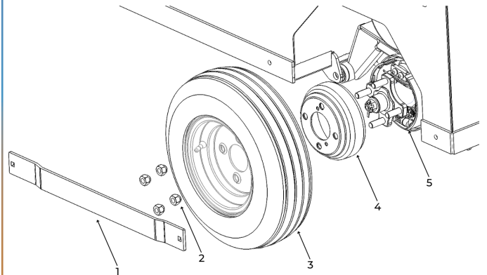
Figure 32. Inspection des freins à tambour.
