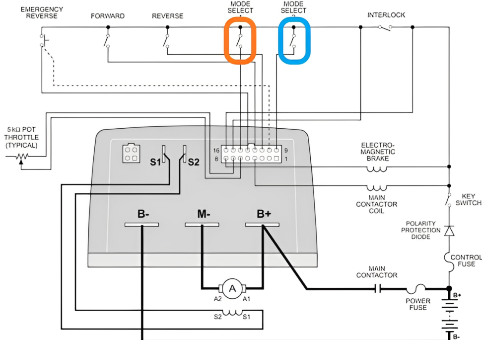
Figure 16. Sélection du mode de conduite.
