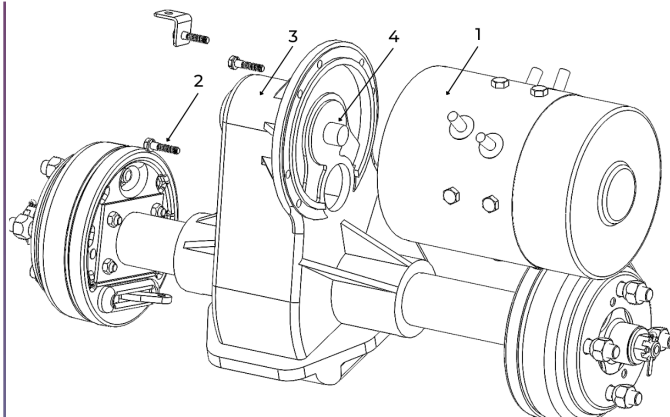
Figure 36. Démontage du moteur.
