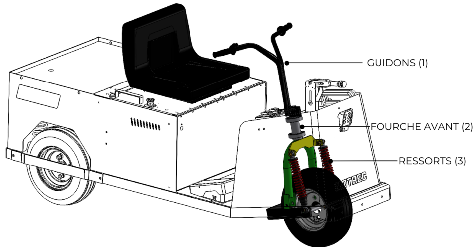
Figure 10. Système de direction.
