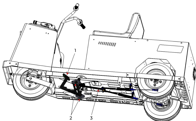
Figure 33. Inspection du système de freinage.
