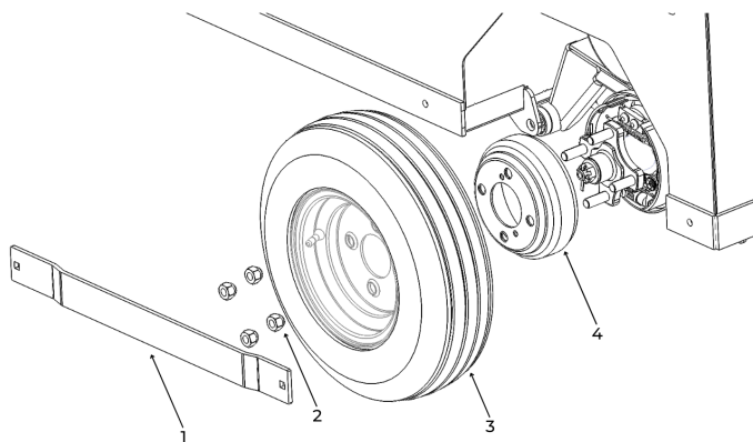
Figure 44. Remplacement des freins à tambour.
