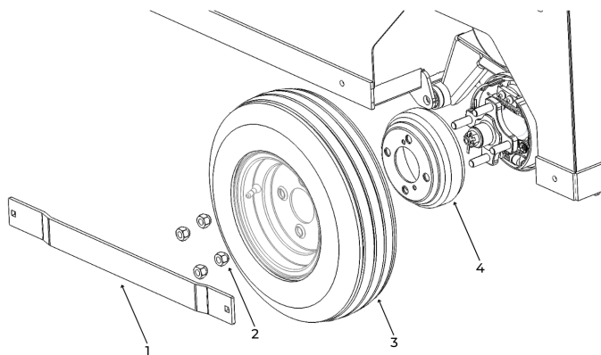
Figure 45. Démontage des freins à tambour.
