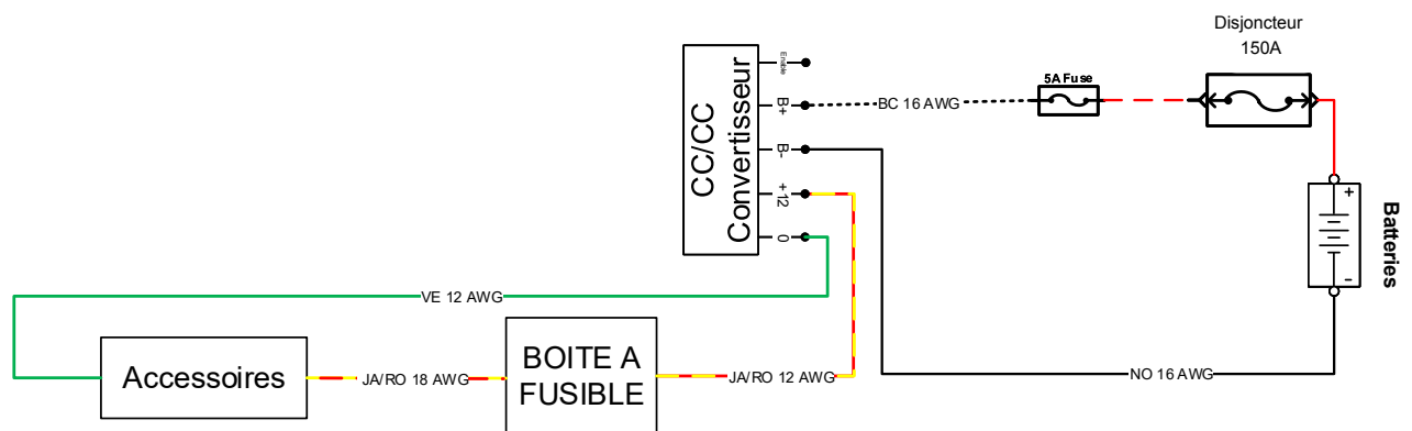
Figure 5. Connexion électrique de l'Énergie Auxiliaire (Annexes 5).
