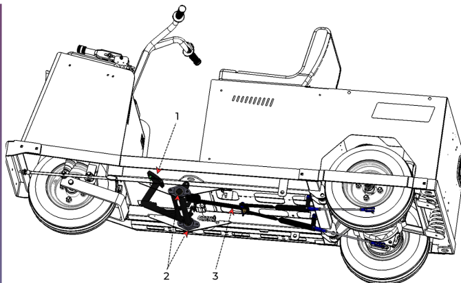
Figure 43. Inspection du système de freinage.
