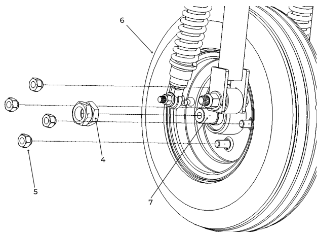
Figure 39. Démontage des roues avant.
