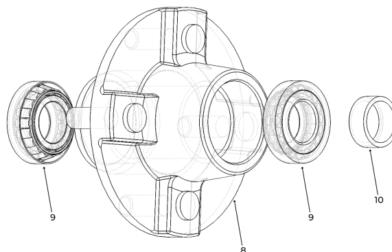
Figure 40. Moyeu de roue avant.
