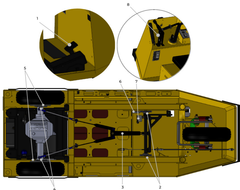
Figure 9. Système de freinage.
