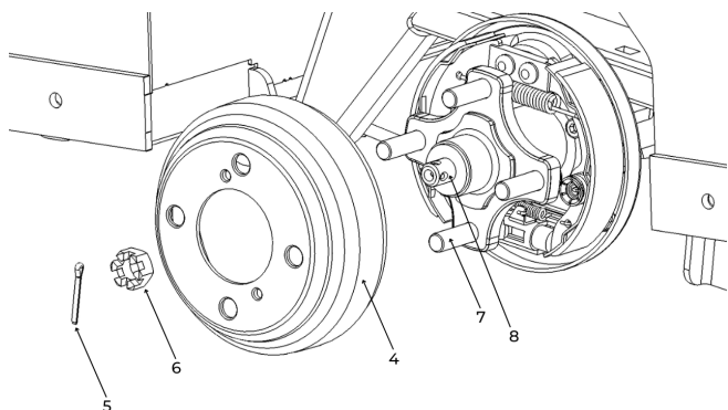
Figure 42 Moyeu arrière.
