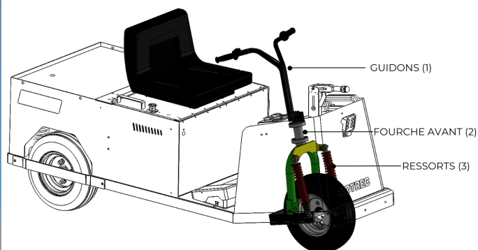
Figure 26. Inspection générale du système de direction.
