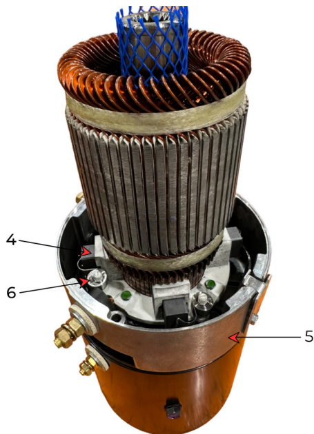
Figure 47. Remplacement des brosses.
