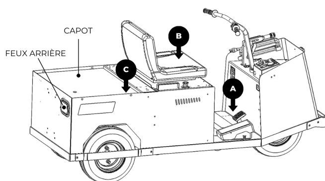
Figure 12. Composants généraux.
