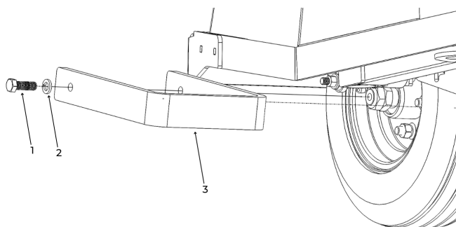
Figure 38. Démontage des roues avant.
