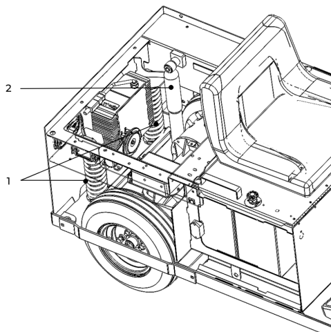
Figure 25. Inspection de la suspension arrière.
