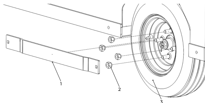
Figure 41. Démontage des roues arrière.
