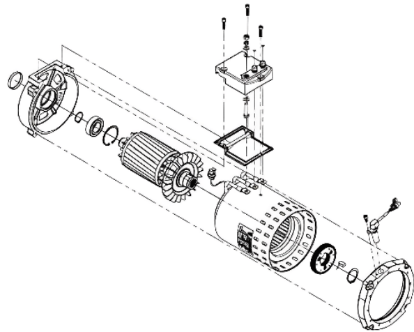
Figure 6. Moteur à Refroidissement Par Ventilateur.
