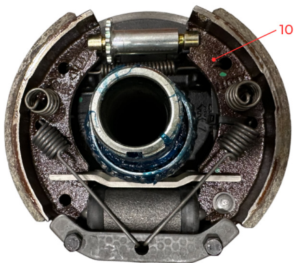
Figure 53. Inspection du système de frein à tambour.
