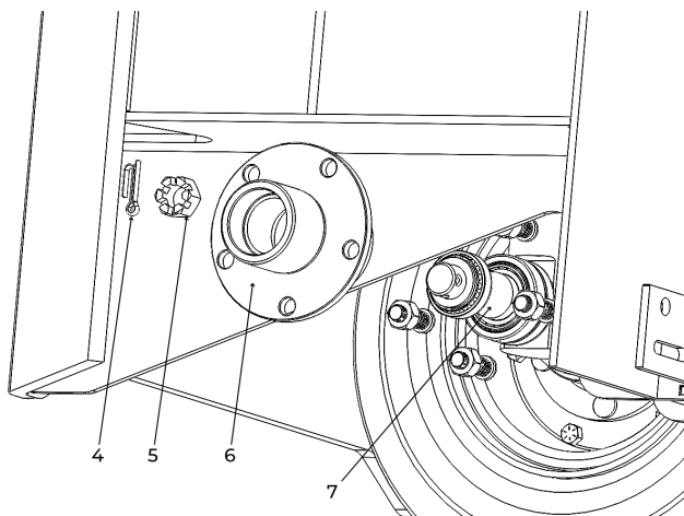
Figure 44. Maintenance du moyeu.
