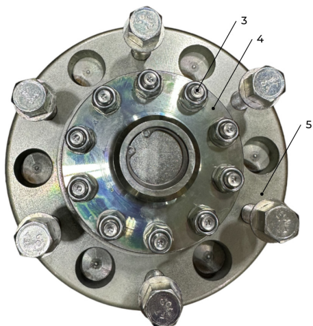
Figure 61. Retrait des boulons et du couvercle du moyeu de l'essieu.
