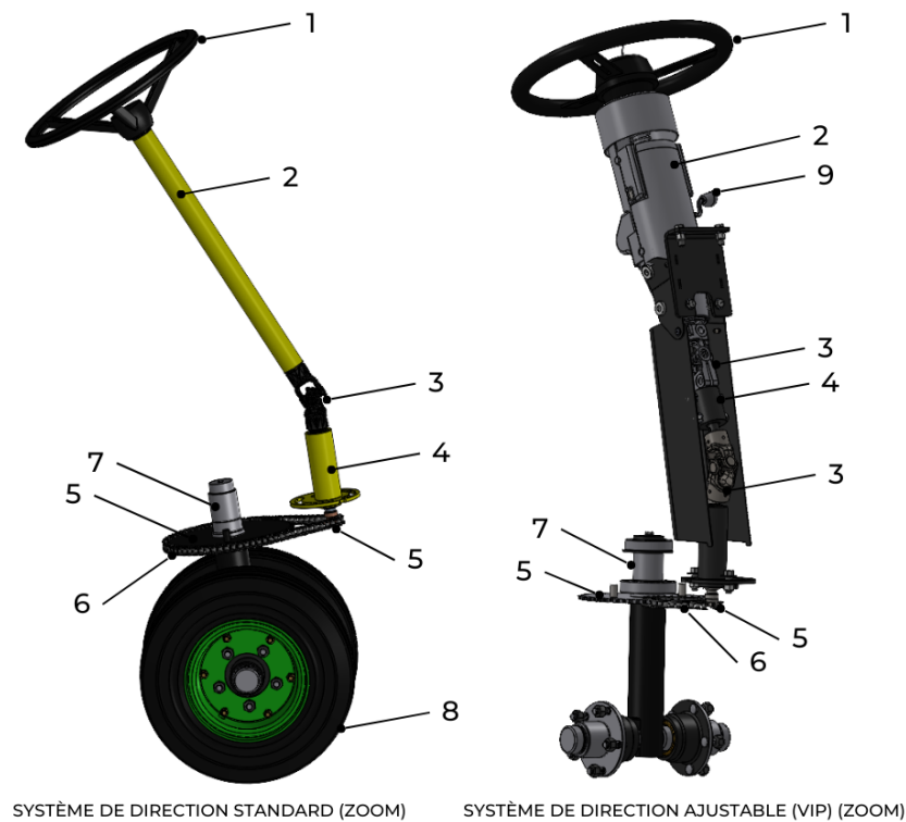
Figure 9. Système de direction.
