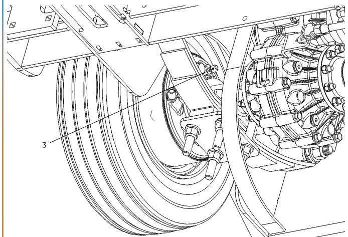
Figure 59. Purge des freins à tambour.
