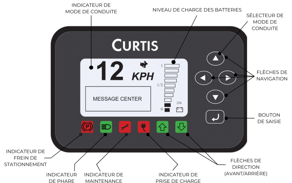
Figure 13. Afficheur.
