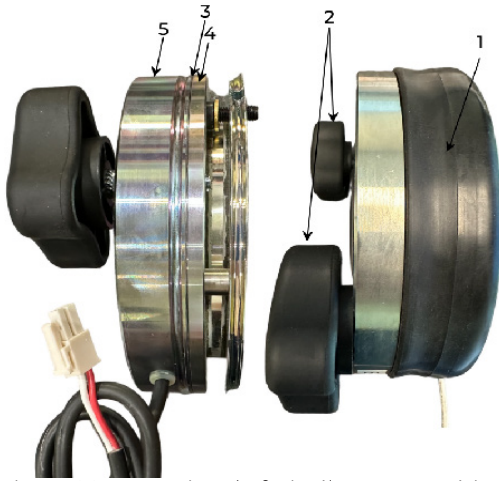
Figure 26. Inspection du frein électromagnétique.
