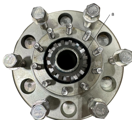
Figure 51. Retrait de la rondelle de blocage.
