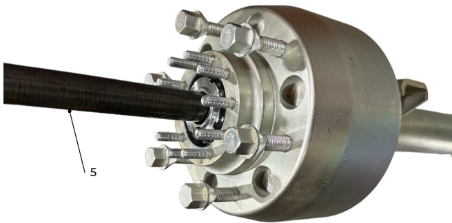
Figure 65. Retrait de l'arbre de l'essieu arrière.
