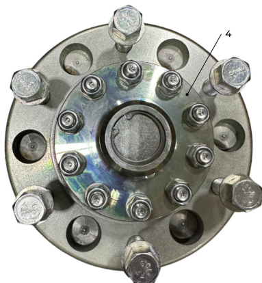
Figure 48. Démontage du couvercle de moyeu d'essieu.
