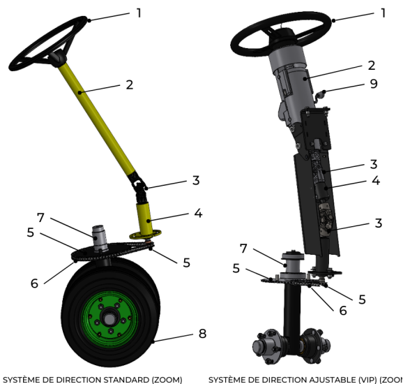
Figure 25. Inspection générale du système de direction.
