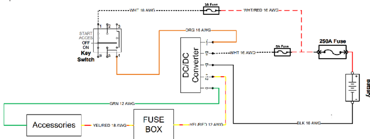
Figure 67. Inspection des bornes d'entrée et de sortie du convertisseur DC/DC.
