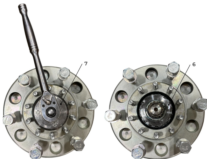
Figure 50. Retrait de l'écrou de blocage.
