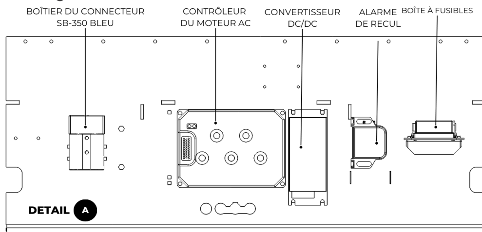
Figure 3. a. Compartiments du Système Electrique Detail A.
