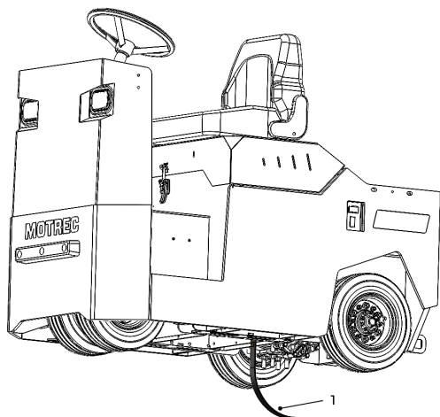
Figure 22. Sangle statique.
