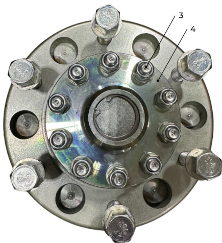
Figure 64. Retrait des boulons et du couvercle du moyeu de l'essieu.
